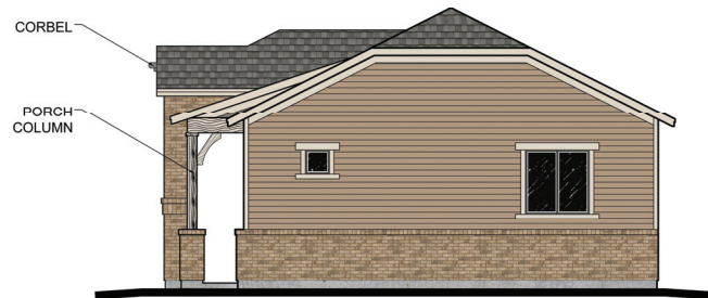
Right Elevation
